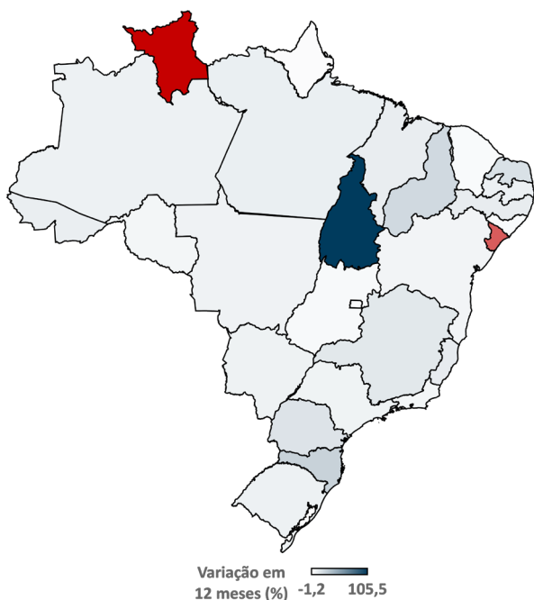
Mapa 3. Variação percentual do número de beneficiários de planos exclusivamente odontológicos por Estado entre Fevereiro/2021 e Fevereiro/2022.
